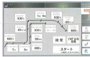
basicモード炉内徐冷設定時
